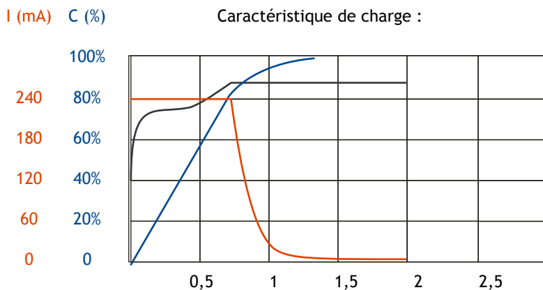
Charge à 240mA Temp. 25±5°C ; RH 60±15%
