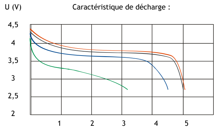
Décharge à 48mA ; RH 60±15%
